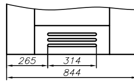
skrzydło SEMPRE „80” ze szczeliną wentylacyjną
