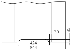
skrzydło SEMPRE „80” z podcięciem wentylacyjnym
