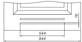
skrzydło VERTIGO „90”, VILANO „90” ze szczeliną wentylacyjną
