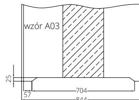
podcięcie wentylacyjne wersja A02-A03 - dopłata 100/123,00
