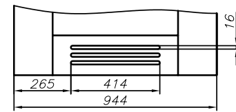
skrzydło SEMPRE „90” ze szczeliną wentylacyjną
