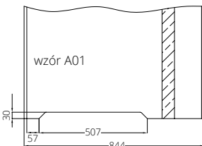
podcięcie wentylacyjne wersja A01 - dopłata 35/43,05
