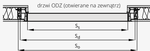
DRZWI OTWIERANE NA ZEWNĄTRZ ODZ
