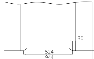
skrzydło SEMPRE „90” z podcięciem wentylacyjnym
