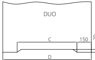
podcięcie wentylacyjne w skrzydłach bezprzylgowych z kolekcji DUO - dopłata 50/61,50
